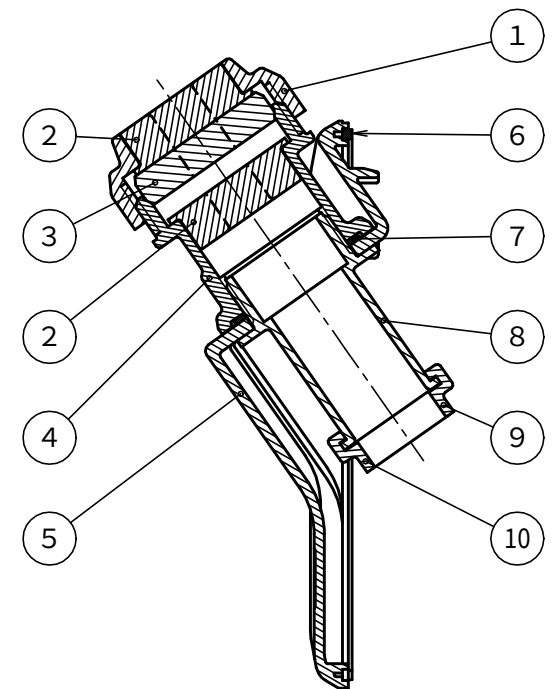
A-A断面図 (1/2)
